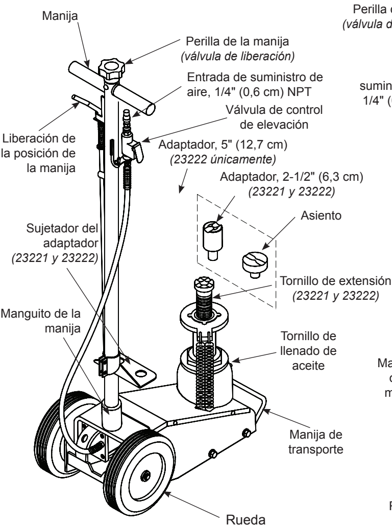
Figura 1: Nomenclatura habitual de un gato para camiones (se muestra 23222)
