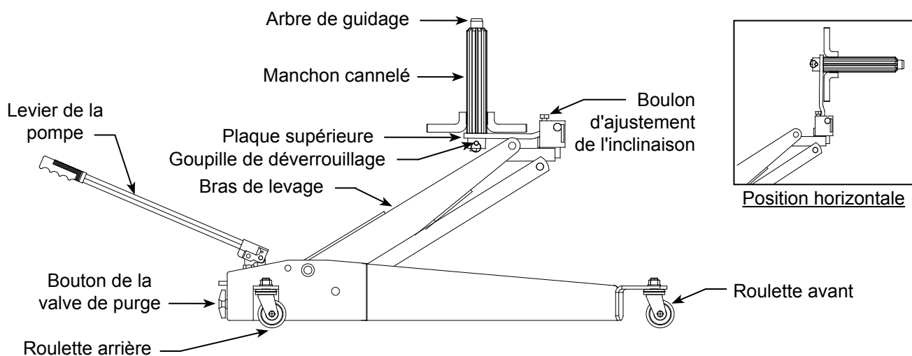
Figure 1 : Composants du modèle 40500
