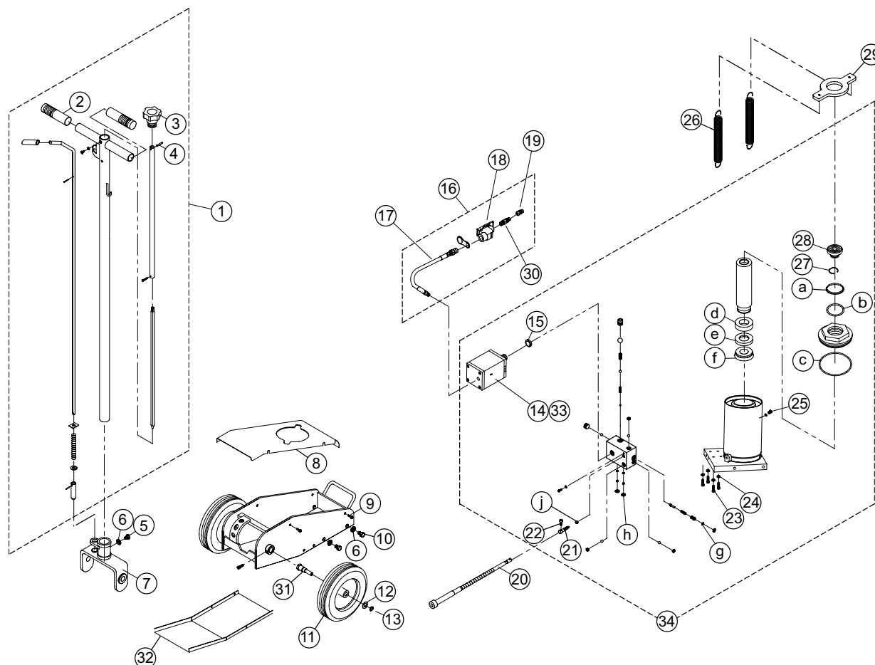
Figure 3 : Illustration des pièces de rechange du modèle BH6301
