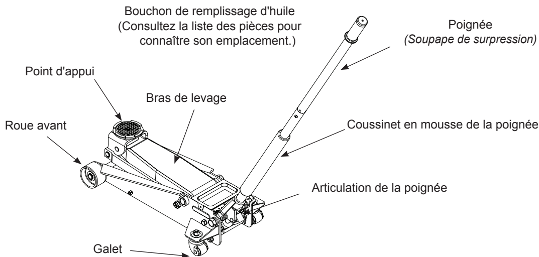
Figure 1 : Pièces d'un cric type
